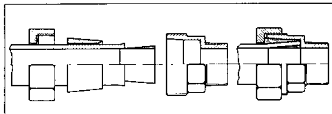
Fig. 21 - Giunto con ancoraggio a tenuta mediante compressione del tubo di PE
