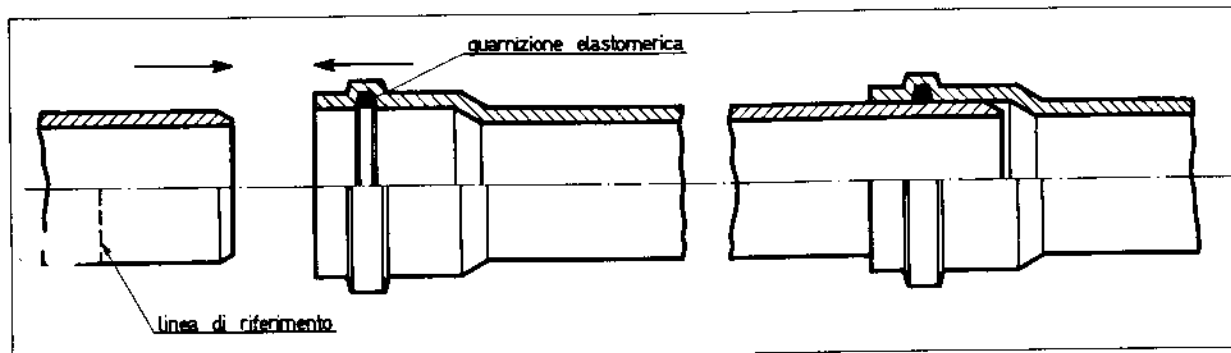
Fig. 4 - Giunto semplice del tipo scorrepolle con guarnizione elastomerica per tubi di PVC
