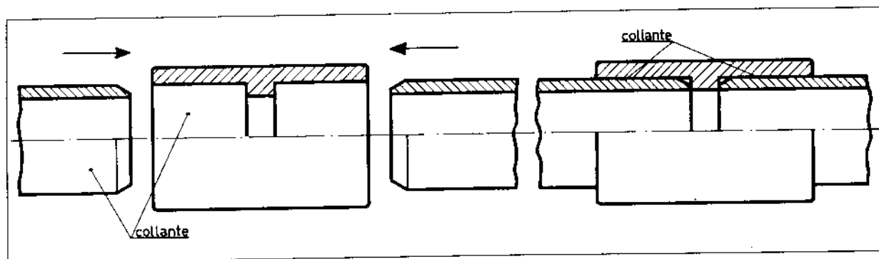
Fig. 2 - Giunto a manicotto del tipo non scorrevole ottenuto per incollaggio per tubi di PVC
