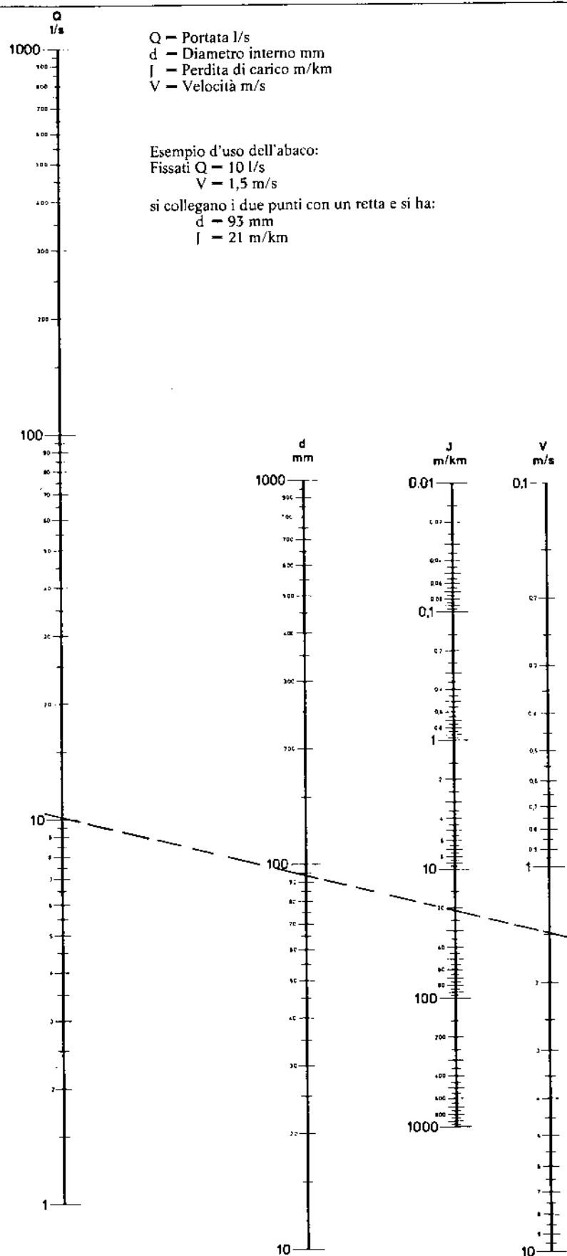
Fig. 9 - Abaco delle perdite di carico nei tubi di PVC rigido, di PE a.d., di PE b.d. ricavato dalla formula di Blasius.
