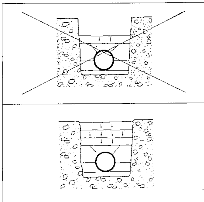
Fig. 12 - Riempiemento dello scavo
