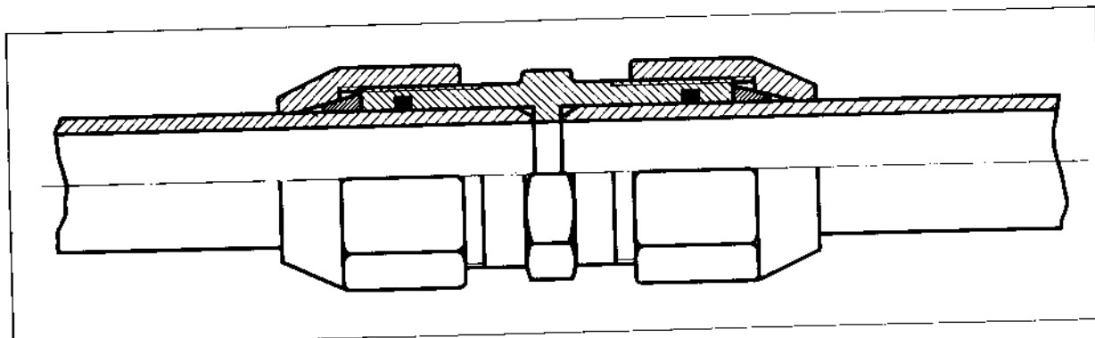
Fig. 6 - Giunto con ancoraggio del tubo di PE mediante anello o ghiera di graffaggio
