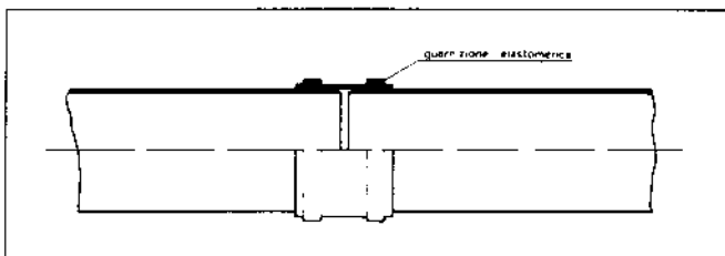
Fig. 18 - Giunto a manicotto del tipo elastico con guarniz. elastom.
