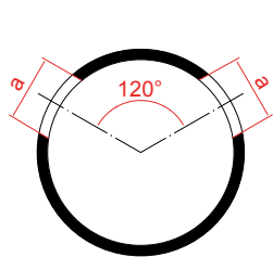
Fessurazione C2
