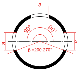
Fessurazione C3
