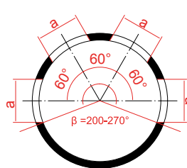
Fessurazione C4
